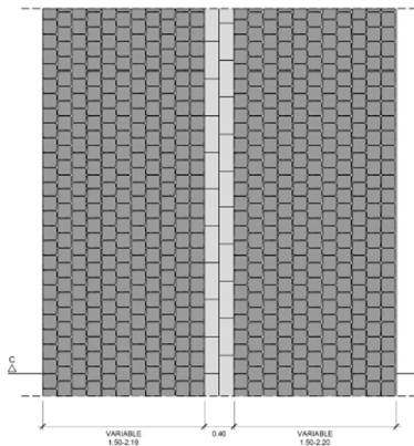
DETALLE PAVIMENTO CALLE MASSANASSA
