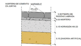
DETALLE A
