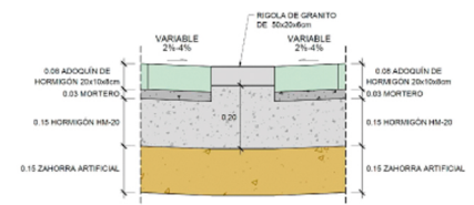
DETALLE C
