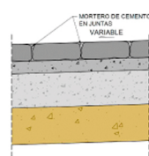
DETALLE C
