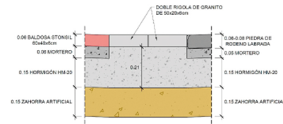
DETALLE B
