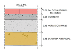
DETALLE A
