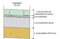
DETALLE B
