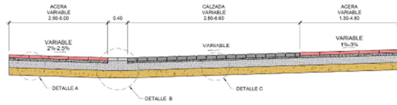
SECCIÓN TIPO A-A PLAZA DE LAS FUENTES
