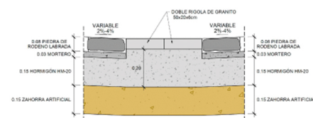
DETALLE B
