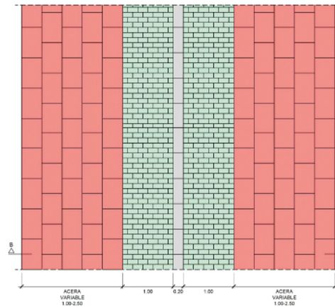
DETALLE PAVIMENTO CALLE SANTO DOMINGO
