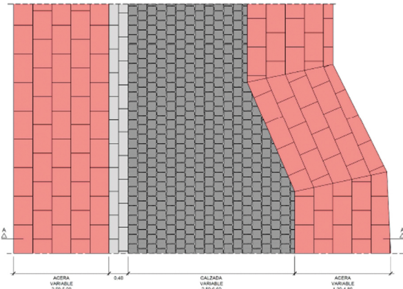
DETALLE PAVIMENTO PLAZA DE LAS FUENTES
