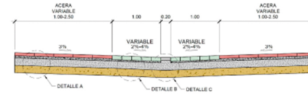
SECCIÓN TIPO B-B CALLE SANTO DOMINGO
