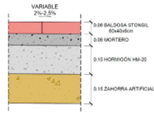
DETALLE A
